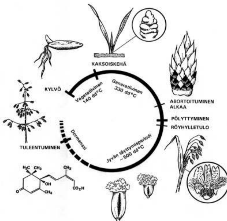
Kuva 5. Viljakasvin elämänsyklin keskeisimmät merkkipaalat ja niiden ajoittuminen Suomen kasvuoloissa tehoisana lämpösommana ilmaistuna. (Kuva: Olli Parkkari)
